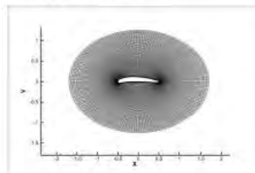
二次元翼
