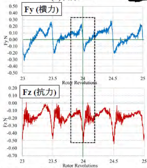
(C) 支持アーム
