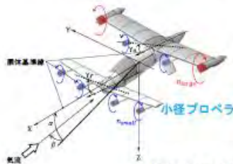
【プロペラの回転方向】
