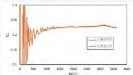
揚力係数CL履歴
