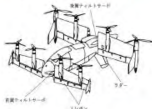
【ホバリング試験その2】
