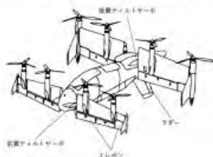
【ホバリング試験その1】
