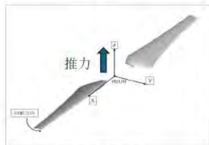
推力の向きと座標系
