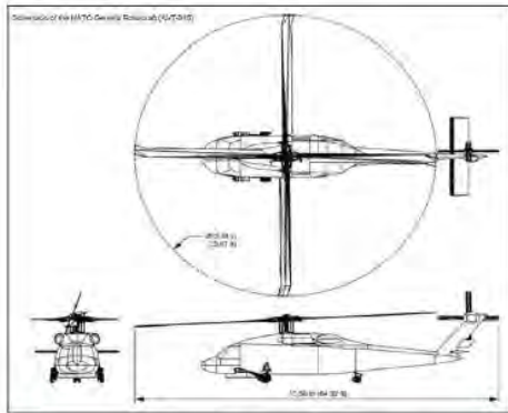
NATO-Generic Rotorcraft諸元
