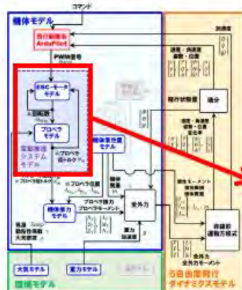
数学モデル (柳原研究室)
